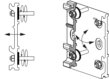
Justierscheibe für präzise Montage der Konsolen
